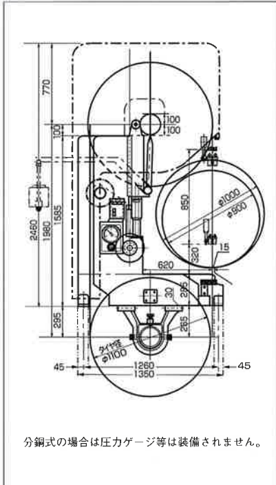
▲HE-1100A型帯鋸盤に定規付テーブル盤を装備(定規付テーブル盤には固定式と回転式があります)
