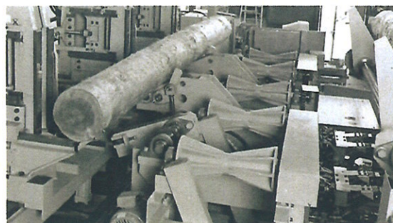
▲ツツミ型ライブローラ Concaved Live Rollers
