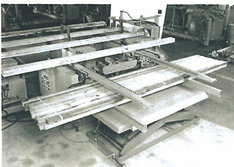
▲テーブルリフター(自動積込装置付結束機) Table Lifter (Automatic Strapping Machine with Products Loading System)
