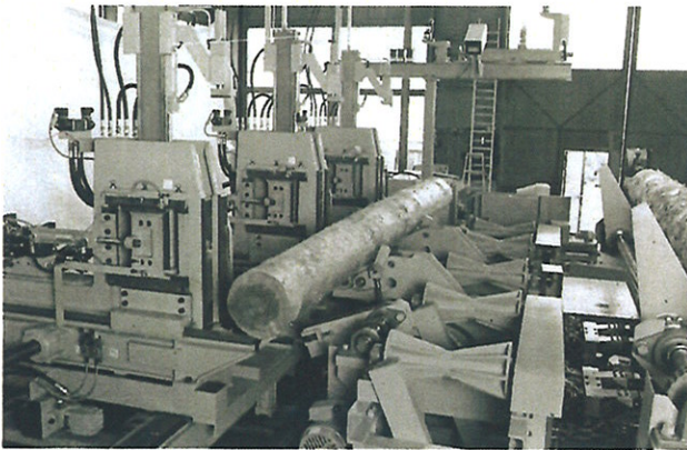
▲送材車用チャージャー装置 Automatic Log Charger for Carriage
