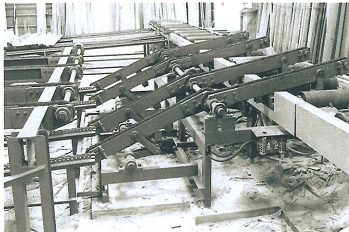
▲ターニングローダ選別スキッド Select Skid (Chain Type) Turning Loader
