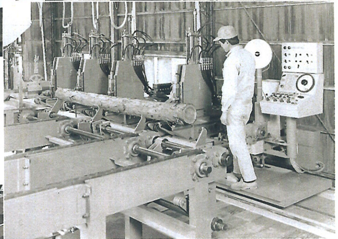
▲HT-008-II型原木搬入盤台 HT-008-II Type;Chain Live Deck
