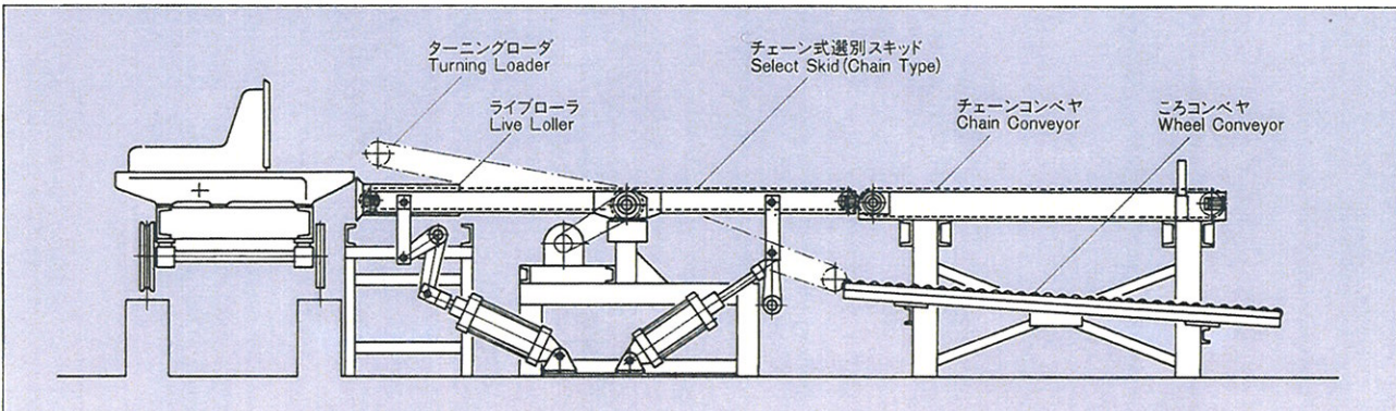
▲ターニングローダ選別スキッド Select Skid (Chain Type) Turning Loader
