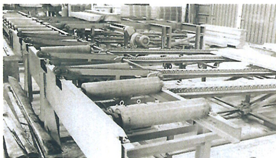
▲ランバーソータ Lumber Sorter
