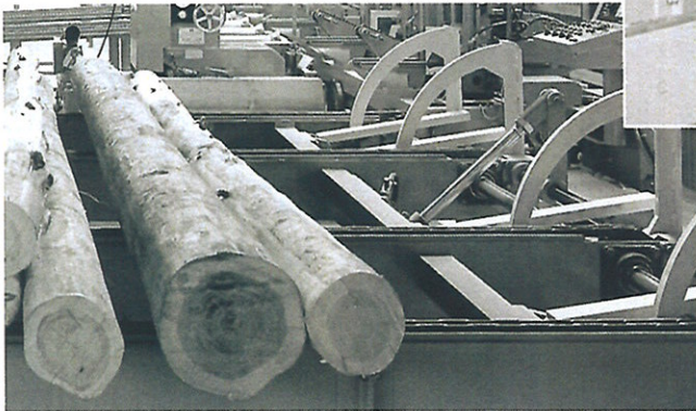
◀HT-008-I型原木搬入盤 HT-008-I Type;Chain Live Deck
