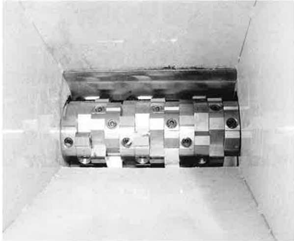
▲ 粉砕メカニズム
